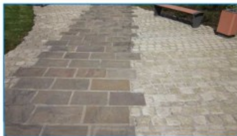
DALLES : Exemple de calepinage
